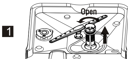
1. Открутите и снимите грубый фильтр
